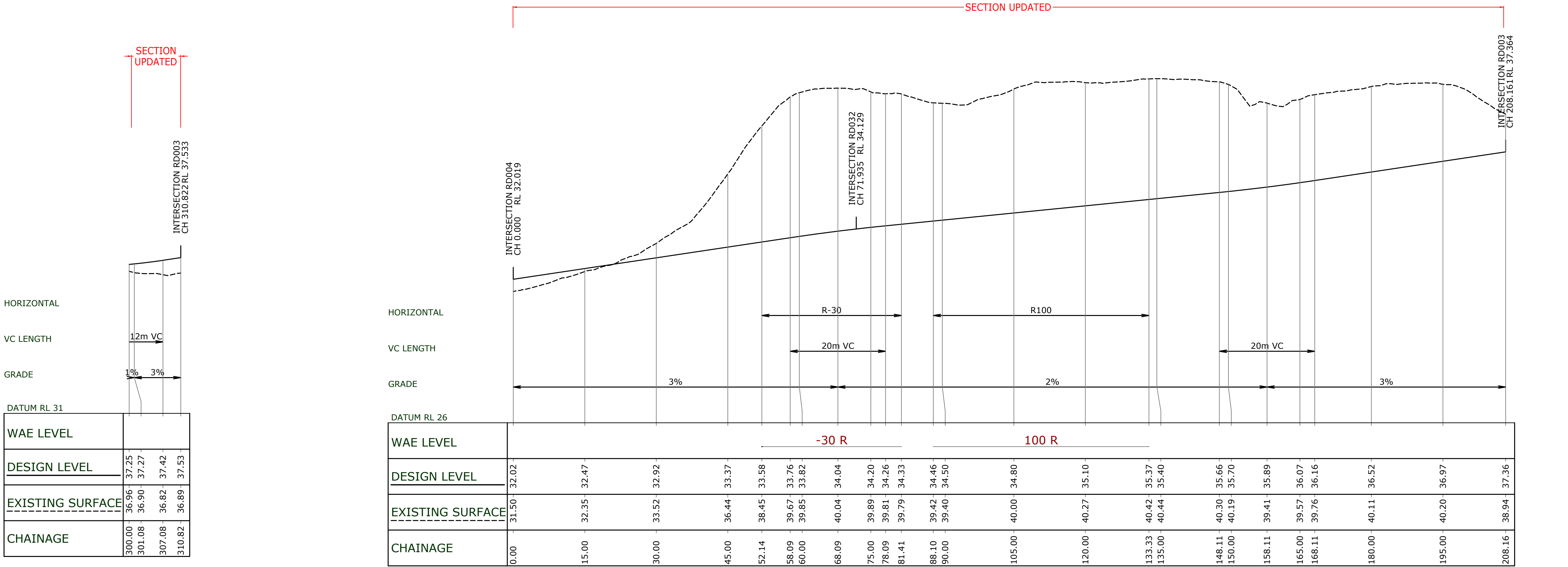
RD030 LONGITUDINAL SECTION 1:500 HORI. 1:100 VERT.
